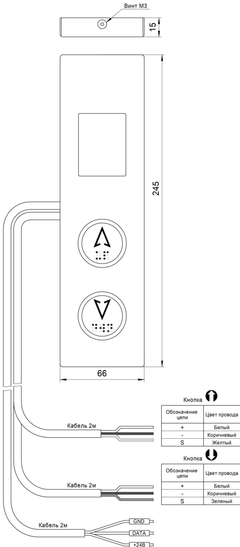
Рис.1 Внешний вид, габаритные и установочные размеры Вызывного поста ВП-2103-1074-09
